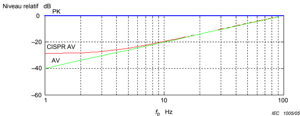
Figure C.1 – Fonction de pondération d'une impulsion de 10 ms pour des détections de valeurs crêtes (PK) et moyennes avec (CISPR AV) ou sans (AV) lecteur crête; avec un contrôleur de période de 160 ms
